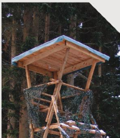
Duża konstrukcja dachowa ▼
